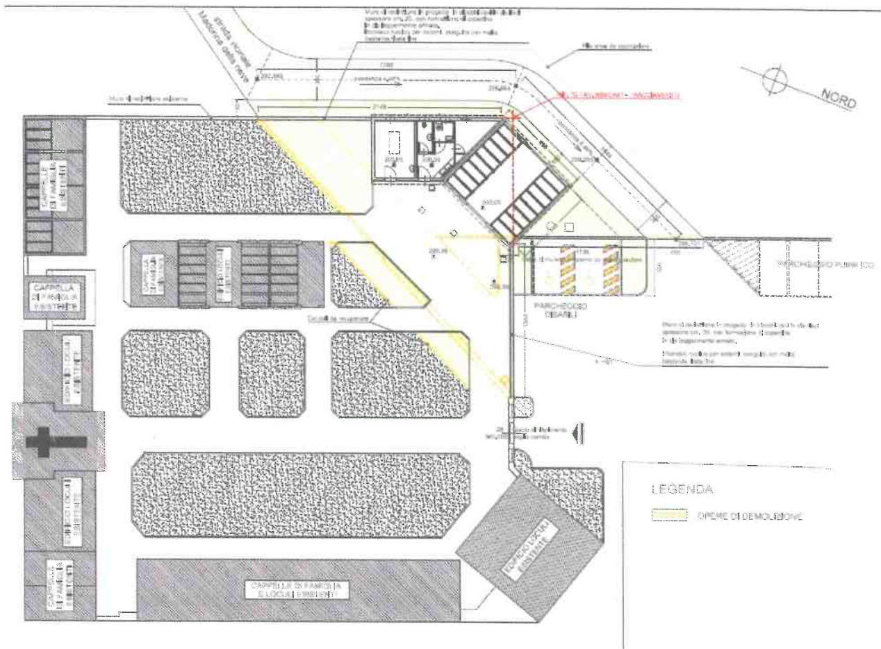
Stralcio planimetria di inquadramento (progetto esecutivo dei lavori)
